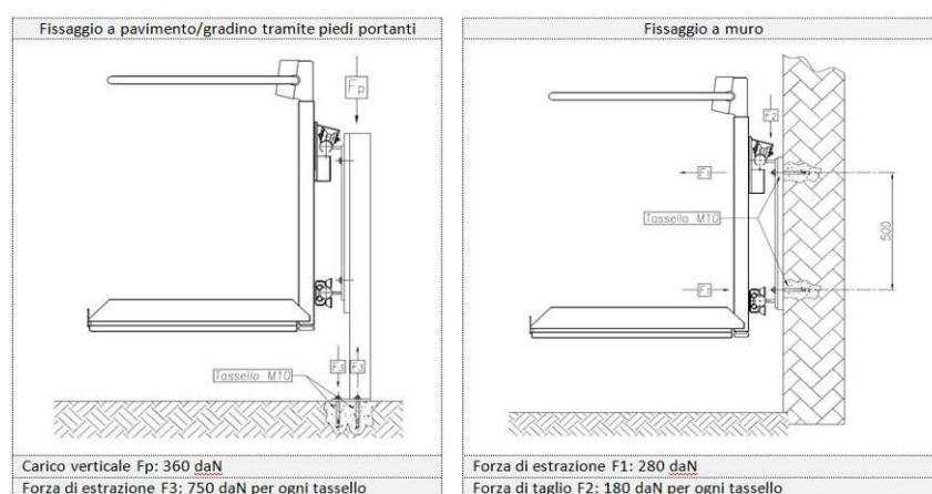
01. Carichi applicati alle strutture alle quali il montacarichi è ancorato, in relazione alla tipologia di fissaggio
